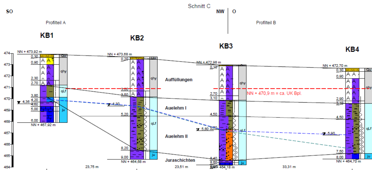
Abb 9. Profilschnitt Bohrprofile nach DIN 4023, Quelle: IGP Geotechnik Pfeiffer GmbH
