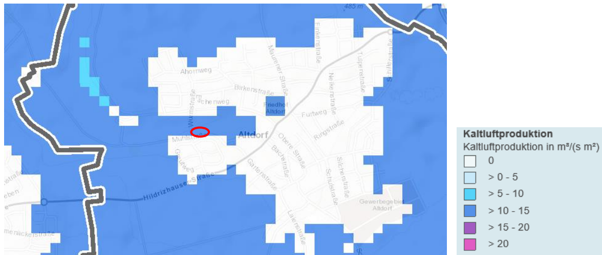
Abb 11. Kaltluftproduktion, Quelle: RegioRISS Verband Region Stuttgart, Plangebiet rot markiert
