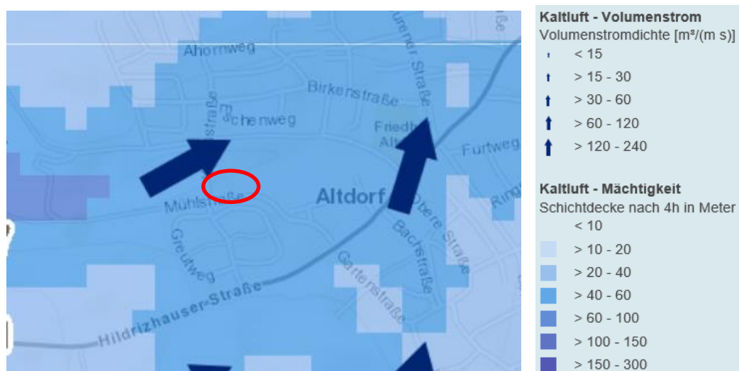
Abb 10. Kaltluftmächtigkeit und Volumenstrom, Quelle: RegioRISS Verband Region Stuttgart, Plangebiet rot markiert
