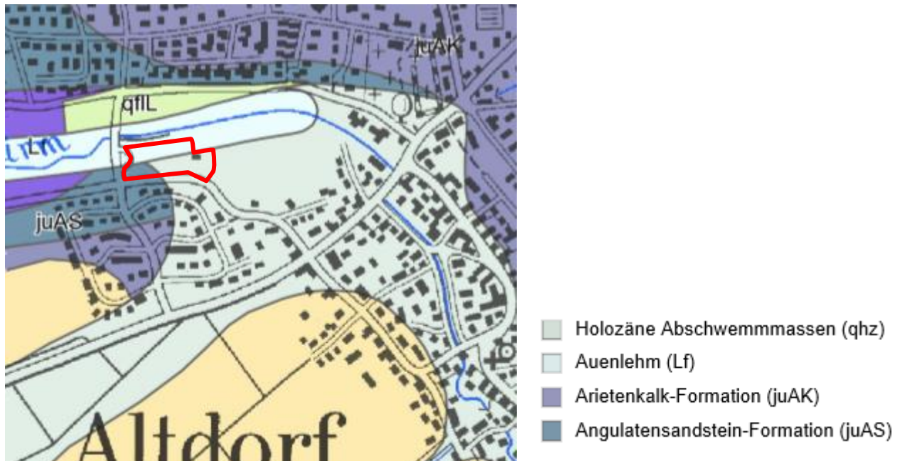
Abb 6. Ausschnitt Geologische Karte GK 50, Quelle: LGRB BW. Plangebiet rot markiert
